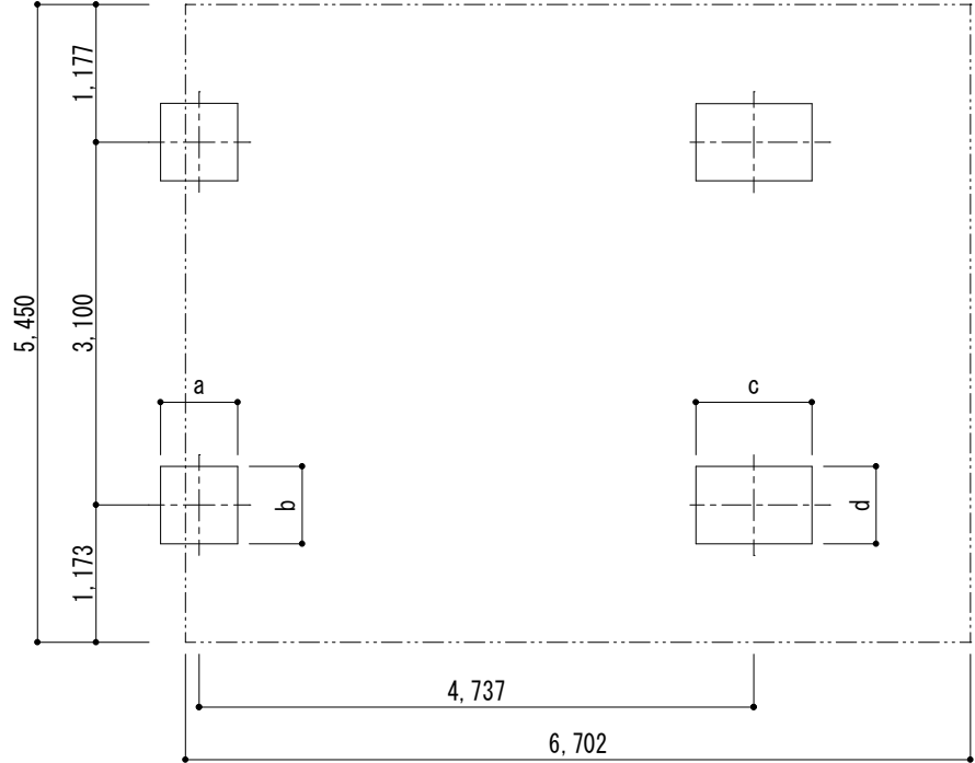
■ 基礎配置図
